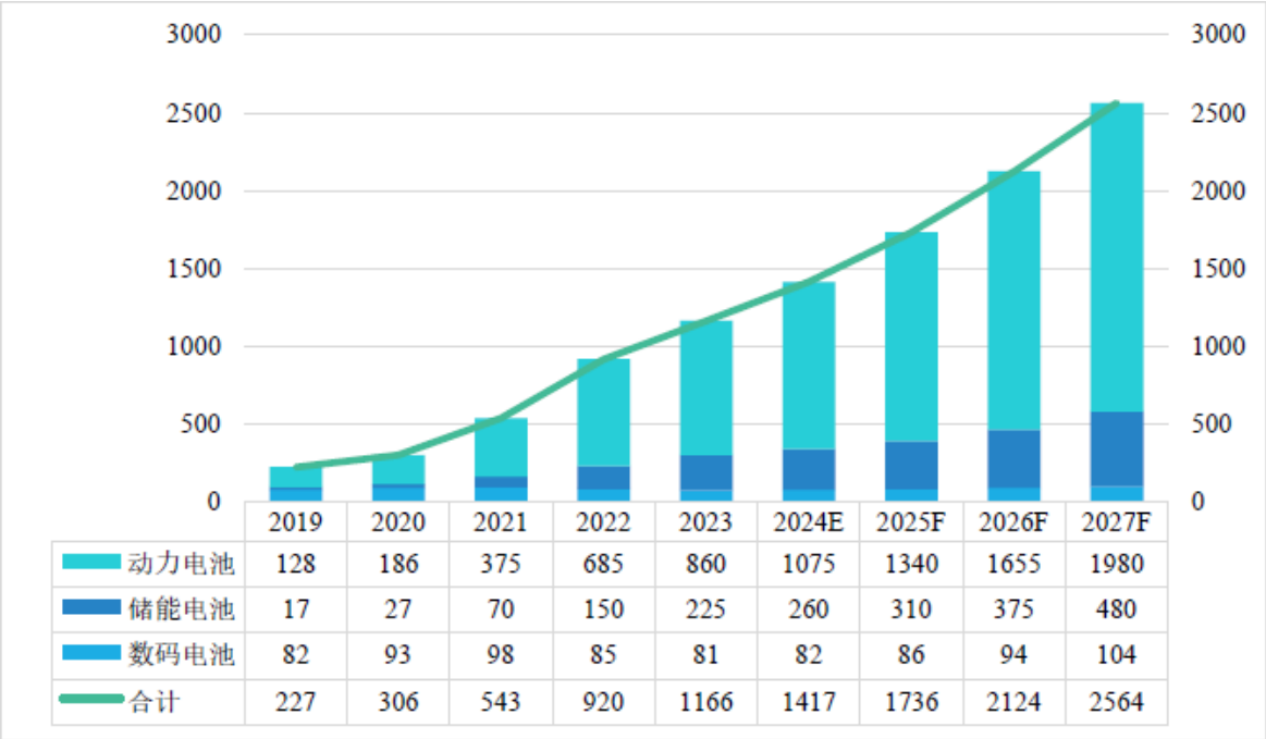
2019-2027 年全球锂电池出货量及预测（GWh）
