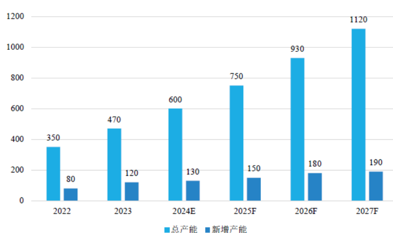
2022-2027 年海外锂电池新增产能及预测 (GWh)
