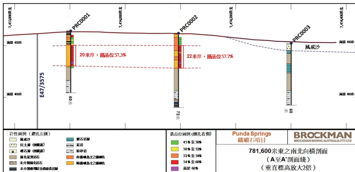
圖3—A至A橫剖面(剖面綫位置見圖2)
