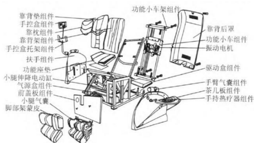
图：按摩椅结构图
