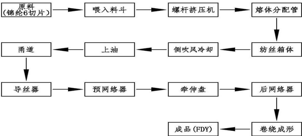
② FDY（全拉伸丝）工艺流程图
