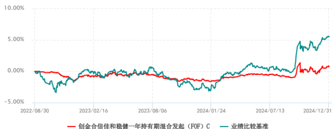
创金合信佳和稳健一年持有期混合发起（FOF）C 累计净值增长率与业绩比较基准收益率历史走势对比图 (2022年08月30日-2024年12月31日)
