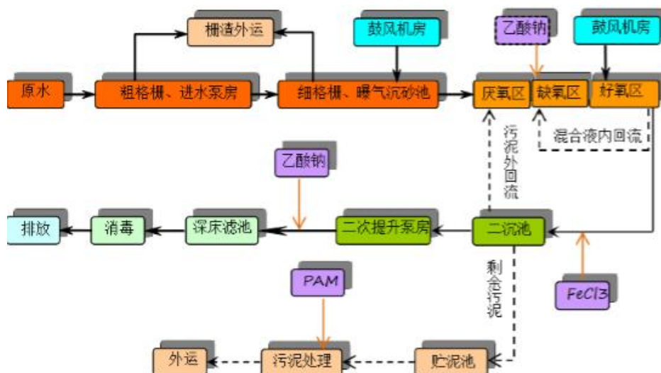
(2) 二期工程工艺流程图
