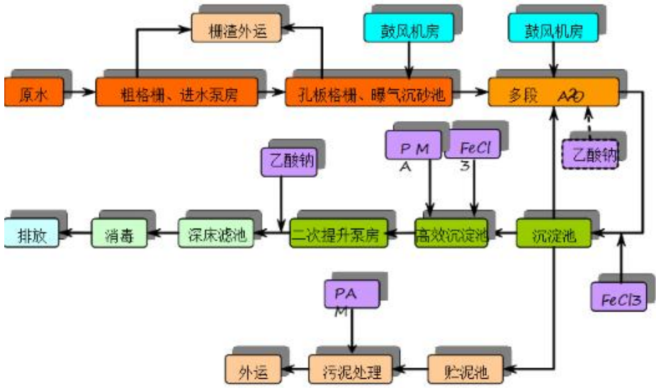
(4) 四期工程工艺流程图
