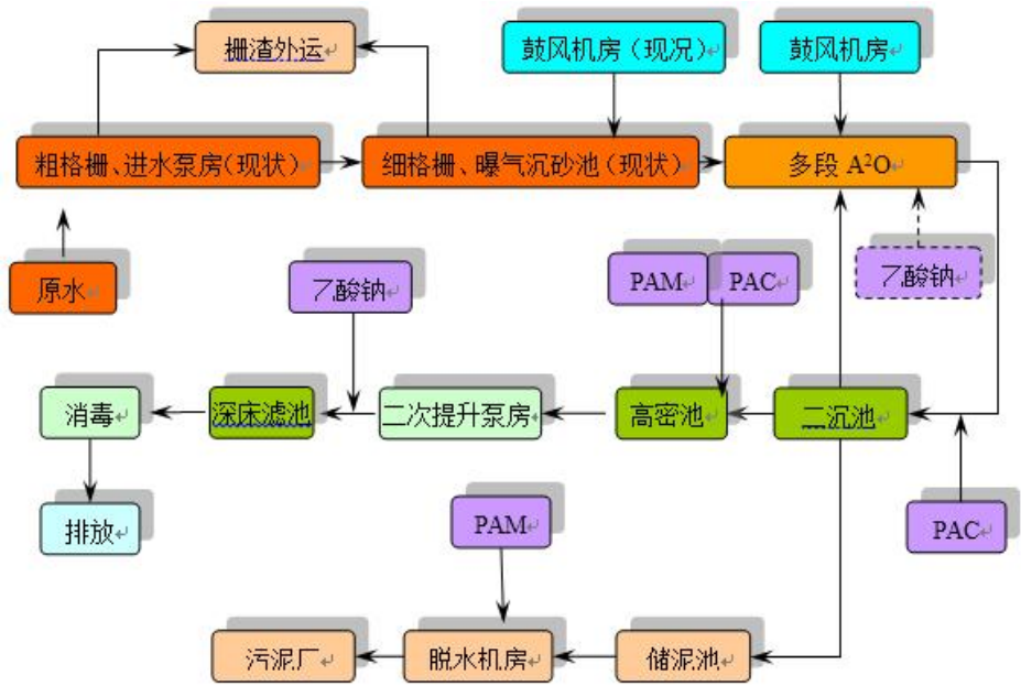
(4) 四期工程工艺流程图
