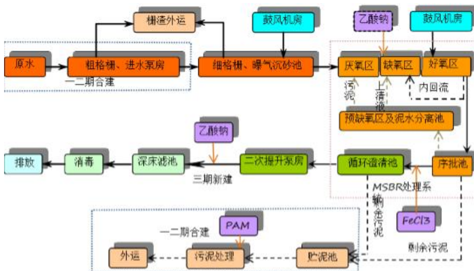
(3) 三期工程工艺流程图
