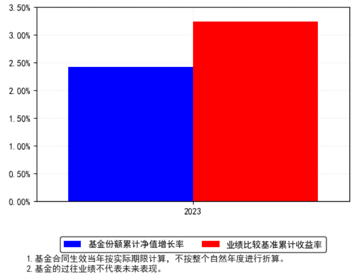
南方浩祥3个月持有债券发起（FOF）每年净值增长率与同期业绩比较基准收益率的对比图（2023年12月31日）
