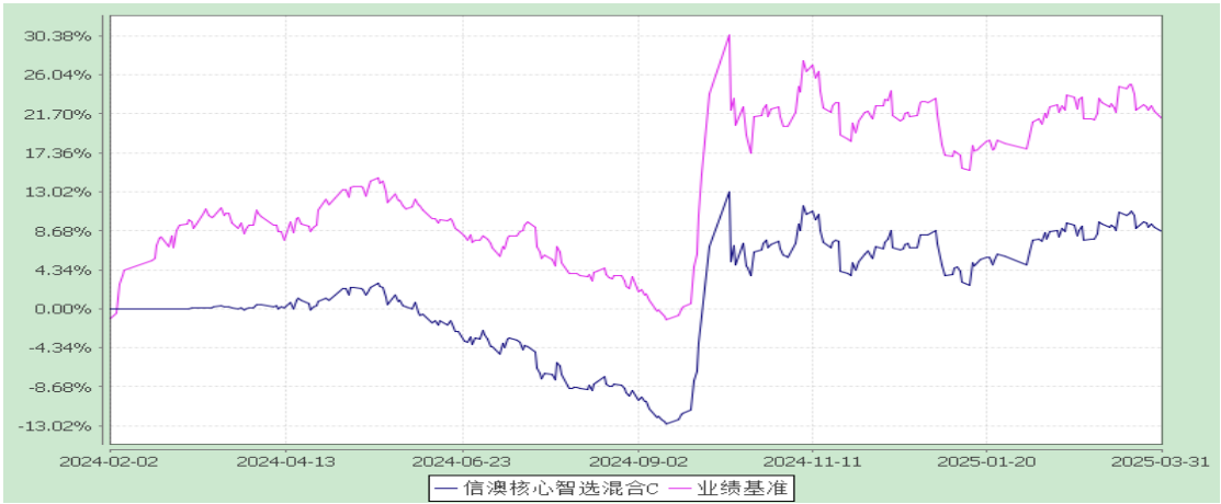
信澳核心智选混合 C 累计净值增长率与业绩比较基准收益率的历史走势对比图 (2024 年 2 月 2 日至 2025 年 3 月 31 日)
