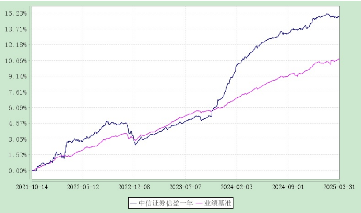
中信证券信盈一年持有期债券型集合资产管理计划 累计净值增长率与业绩比较基准收益率历史走势对比图 (2021 年 10 月 14 日至 2025 年 3 月 31 日)
