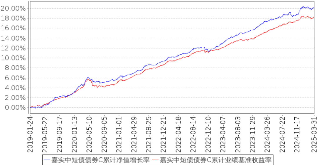
嘉实中短债债券C累计净值增长率与同期业绩比较基准收益率的历史走势对比图 (2019年01月24日至2025年03月31日)
