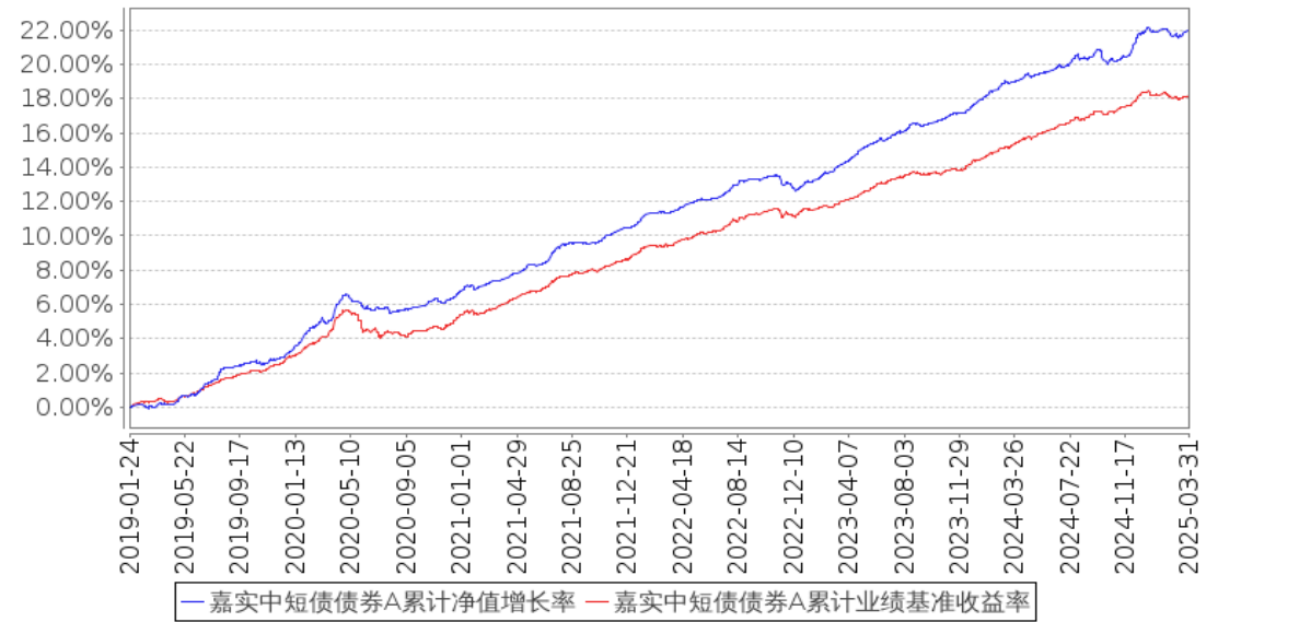
嘉实中短债债券A累计净值增长率与同期业绩比较基准收益率的历史走势对比图 (2019年01月24日至2025年03月31日)
