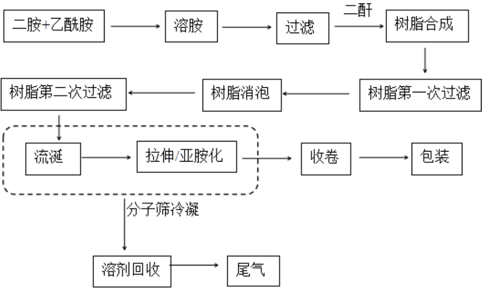
2、聚酰亚胺薄膜 F46 胶带工艺流程图
