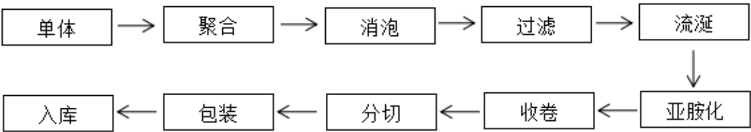
4、双轴定向法制膜工艺流程图
