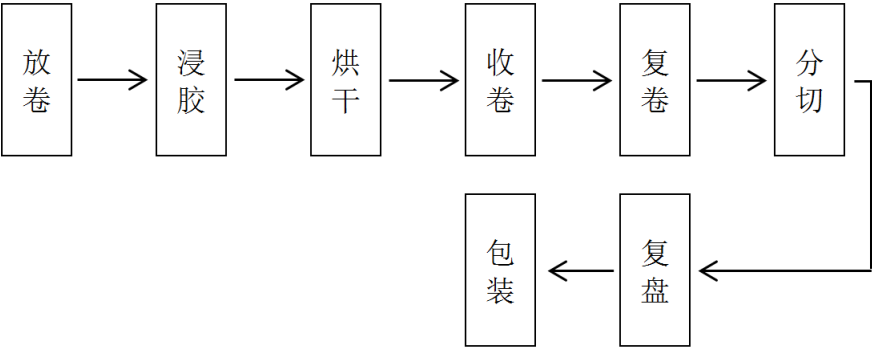
2、聚酰亚胺薄膜 F46 胶带工艺流程图
