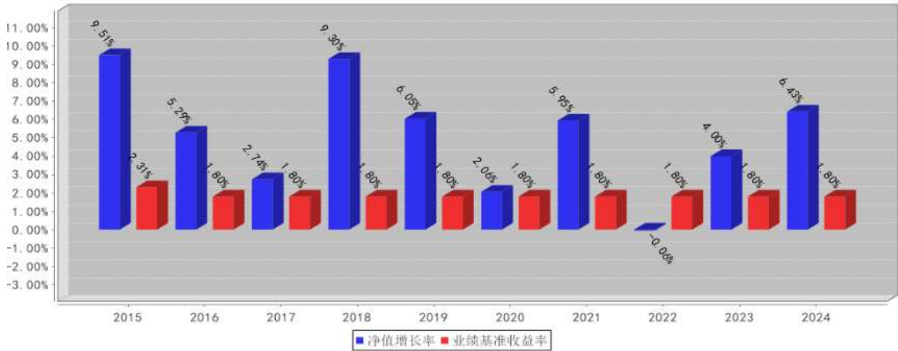
大摩18个月定期开放债券C基金每年净值增长率与同期业绩比较基准收益率的对比图（2024年12月31日）
