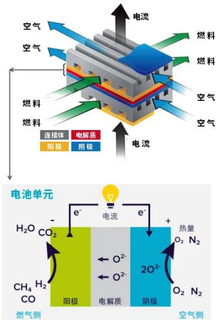
SOFC电池单元工作原理示意图
