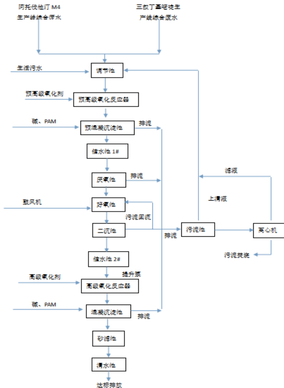
厂区污水处理工艺流程图
