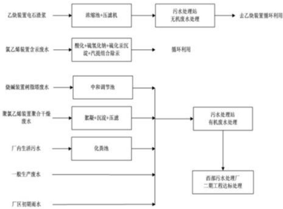
图 2.1-6 全厂废水排放去向图
