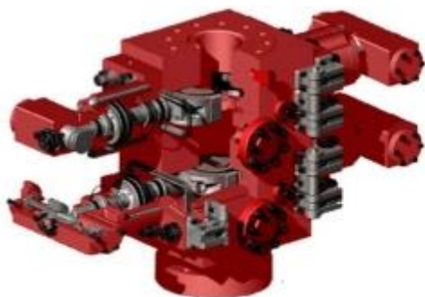
油田防喷器控制装置
