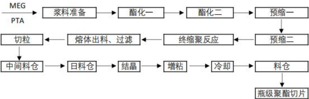
②PTA 工艺流程图
