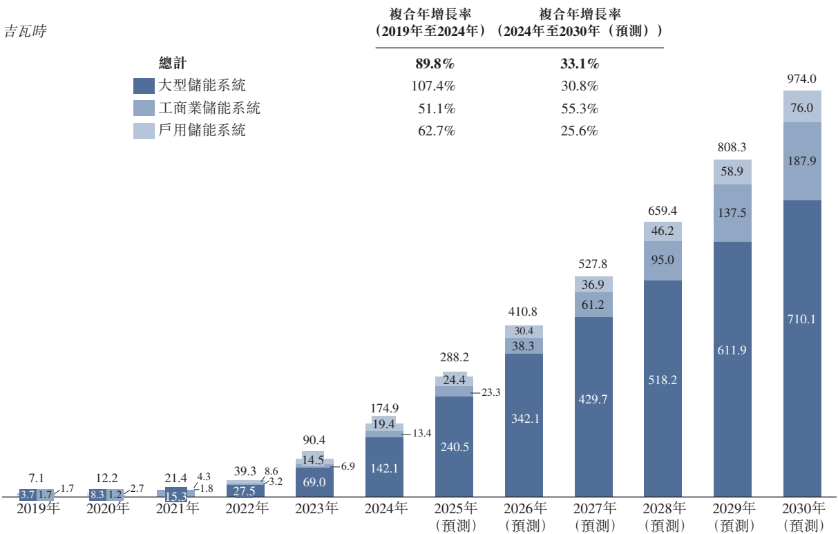
全球儲能系統新增裝機容量 (2019年至2030年(預測))
