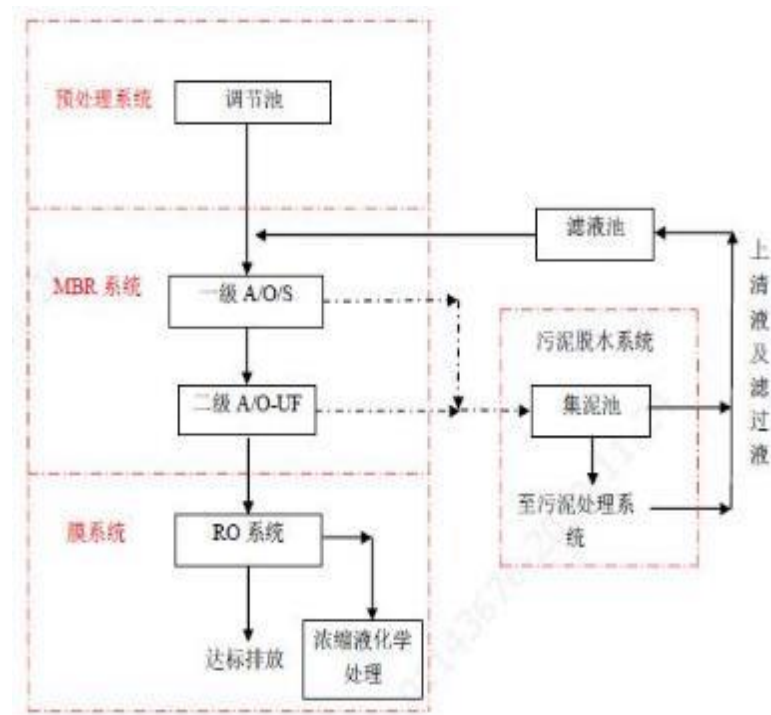
图：填埋场垃圾渗滤液处理工艺流程
