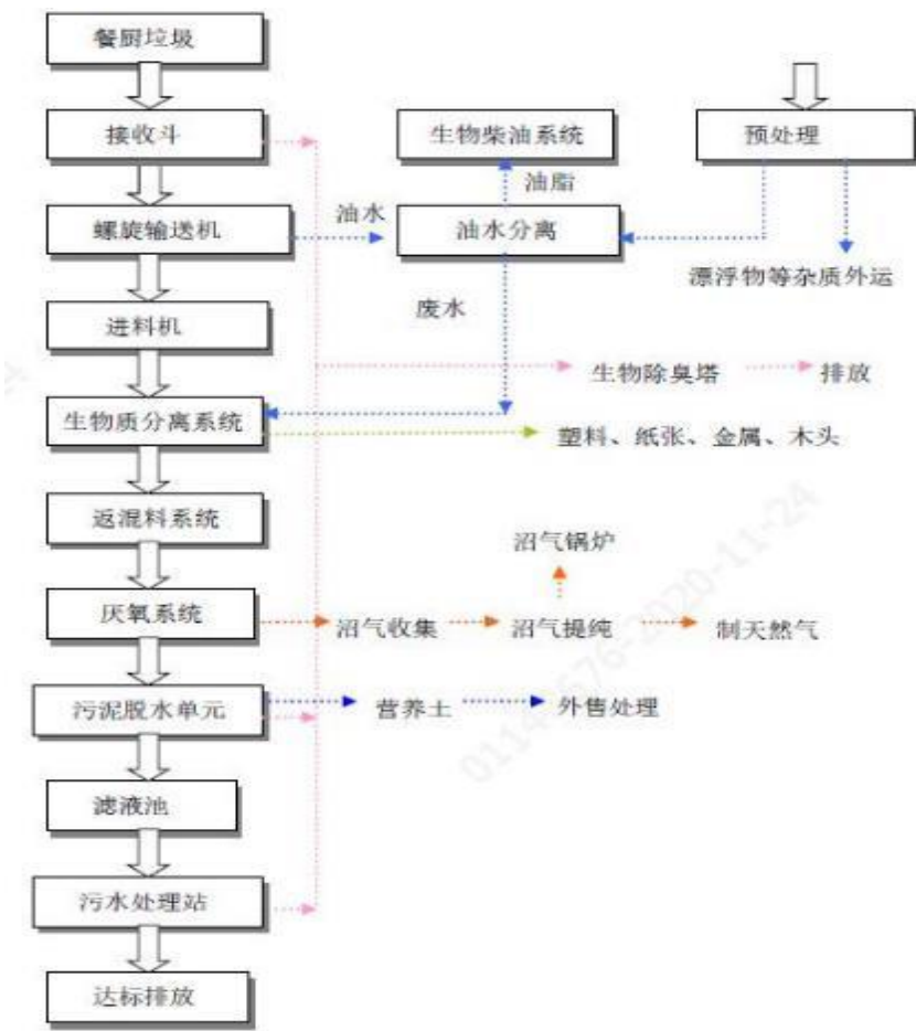
图：餐厨垃圾处理工艺流程
