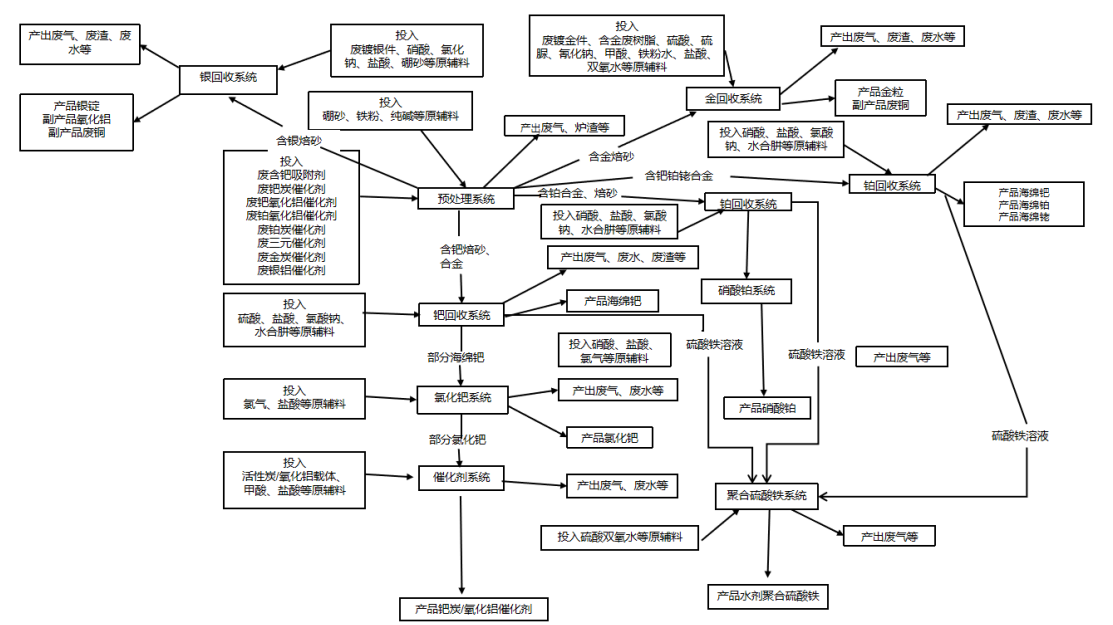
4) 钯、铂、铑、金工艺流程图
