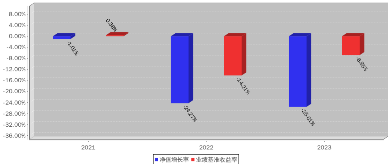
宝盈优质成长混合C基金每年净值增长率与同期业绩比较基准收益率的对比图（2023年12月31日）
