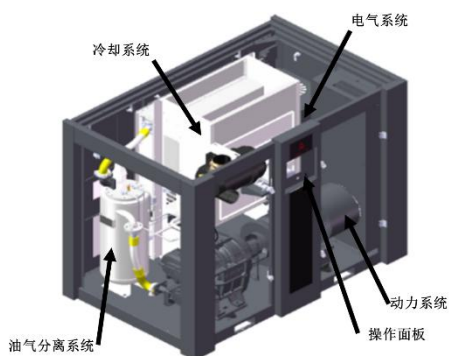
电机驱动螺杆机
