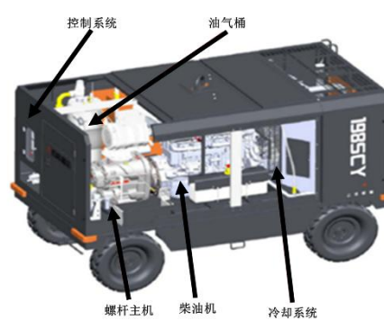
柴油机驱动螺杆机
