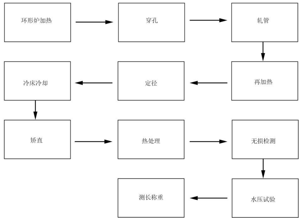
图：华菱阳钢主要生产工艺流程总图
