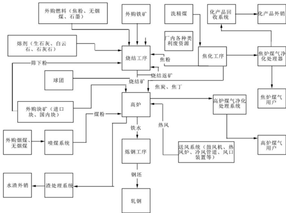
图：华菱湘钢主要生产工艺流程总图
