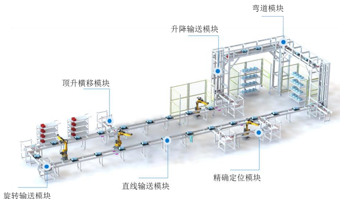
公司模块化输送系统示意图
