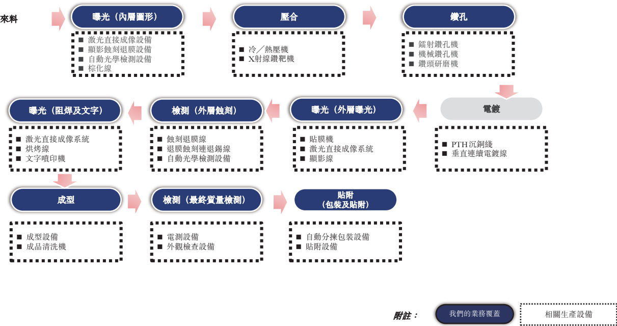
PCB主要生產工序及所需設備
