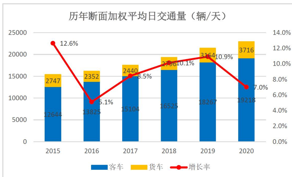
图 16-2 历史断面加权平均日交通量
