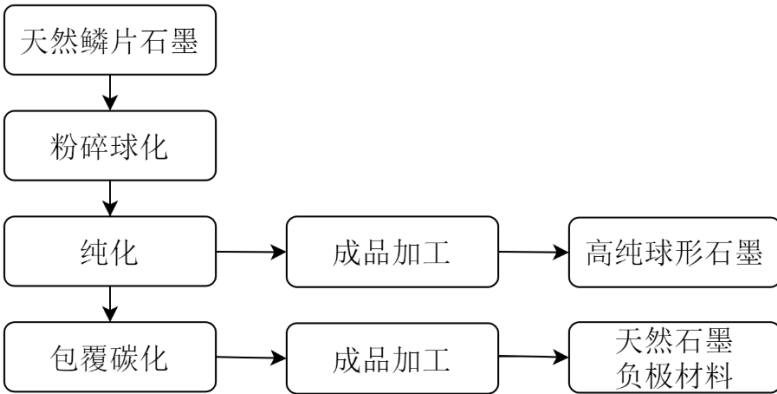
公司天然石墨负极材料生产的主要工艺说明如下：
