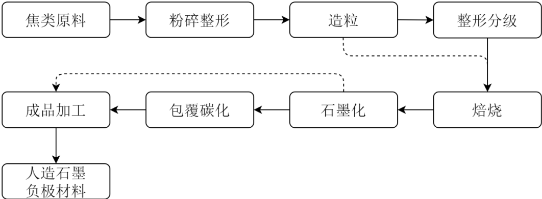
公司人造石墨负极材料生产的主要工艺说明如下：
