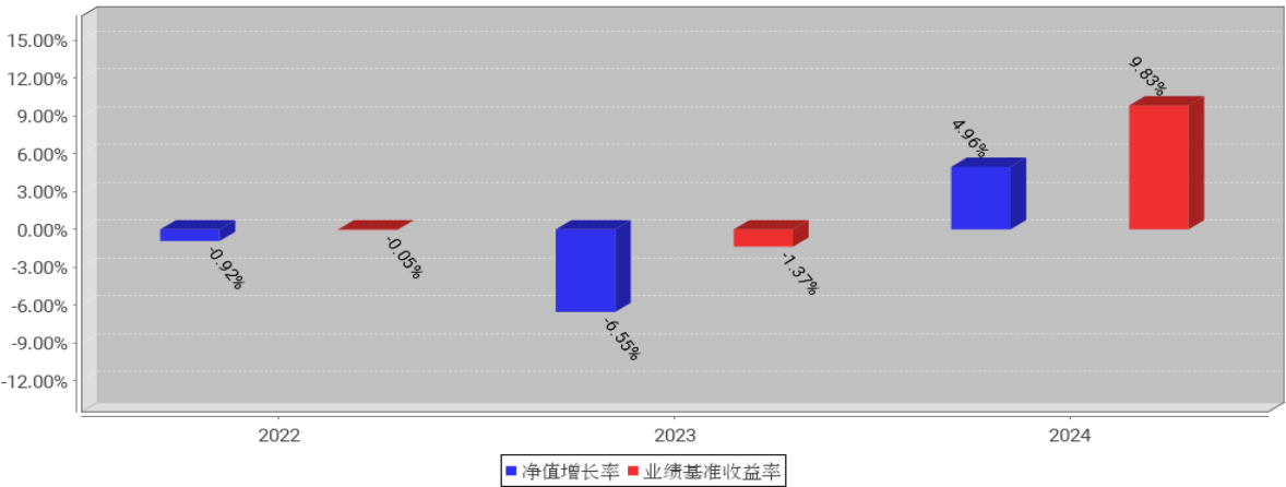
工银养老2035Y基金每年净值增长率与同期业绩比较基准收益率的对比图（2024年12月31日）
