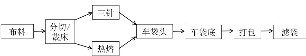
图：制袋生产工艺流程图
