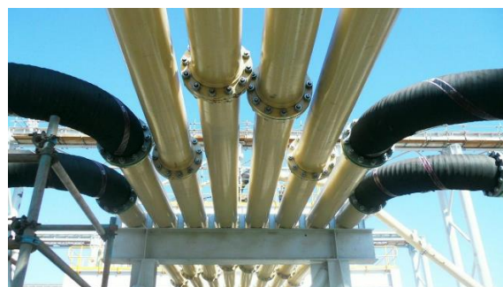
钢橡复合管
