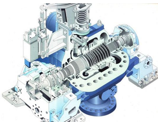
图 1：背压式反动式汽轮机
