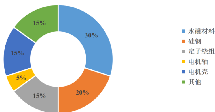
永磁同步电机成本构成
