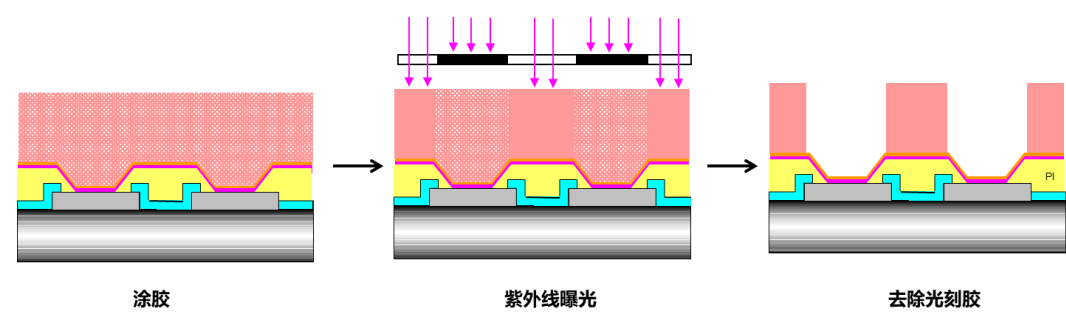
光刻图转移步骤示意图
