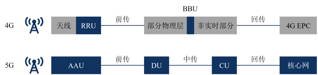
移动通信基站结构
