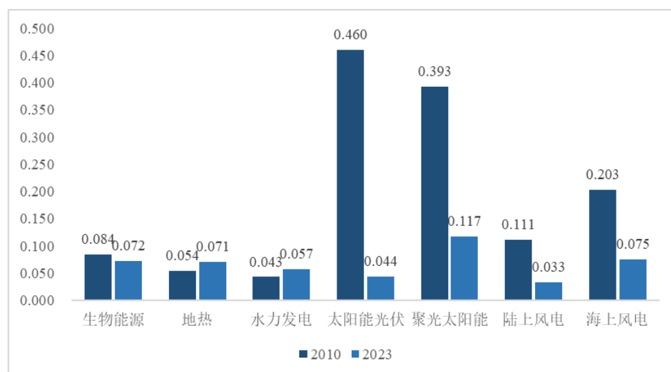
主要可再生能源平准化度电成本（美元/千瓦时）
