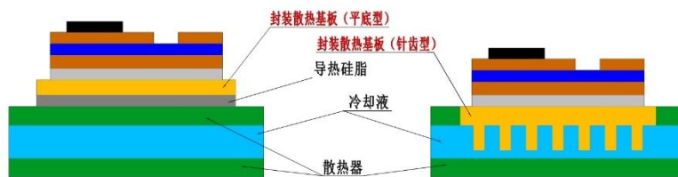
图：采用平底型封装散热基板（左）和针齿型封装散热基板（右）的 IGBT 结构截面图
