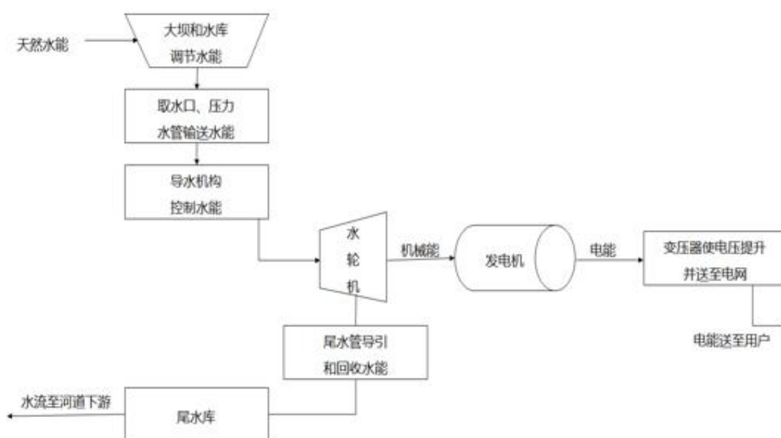
图 14-3：水力发电流程图
