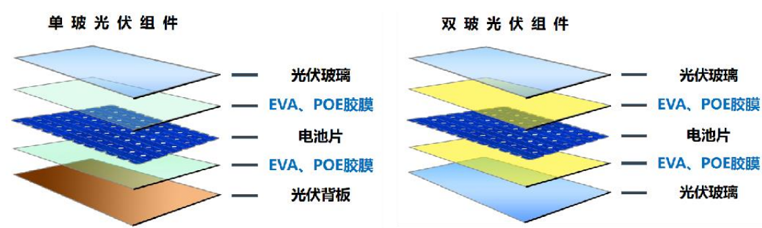
图：单/双玻组件结构示意图
