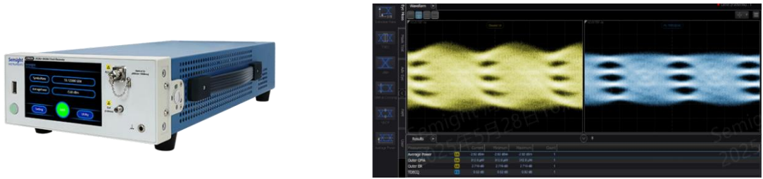
图：时钟恢复单元 图：时钟信号经时钟恢复单元提取前后的眼图对比
