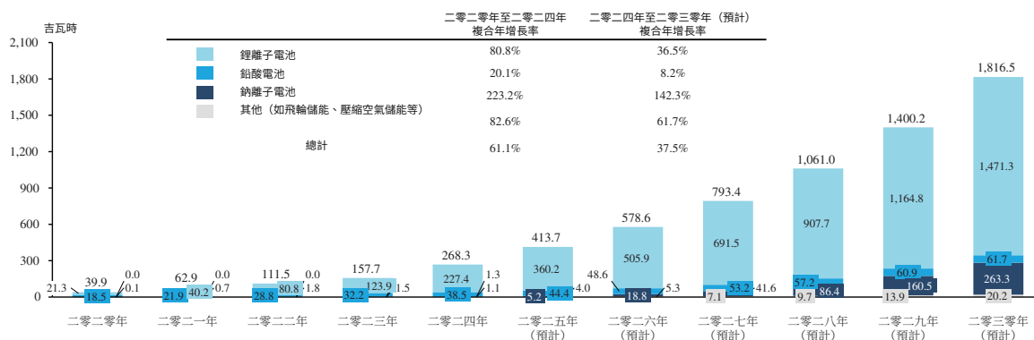
二零二零年至二零三零年(預計)全球儲能新增裝機容量及儲能技術分佈
