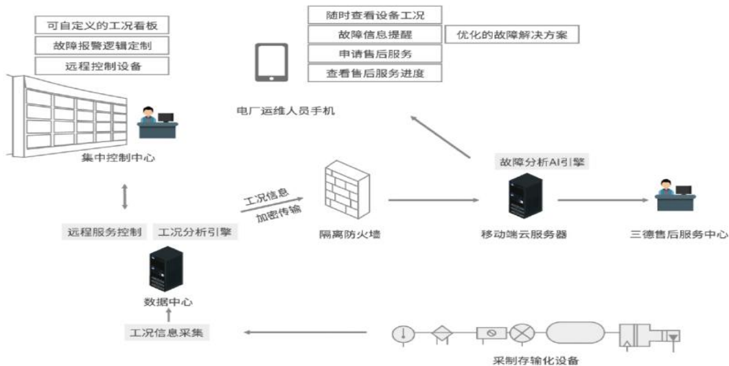
图 4 公司 SDRSS 运维保障系统拓扑图
