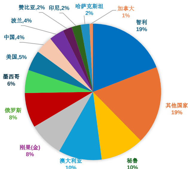
2024 年全球铜矿储量分布
