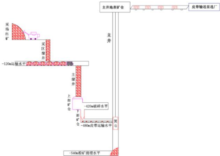
地下采矿生产工艺流程示意图
