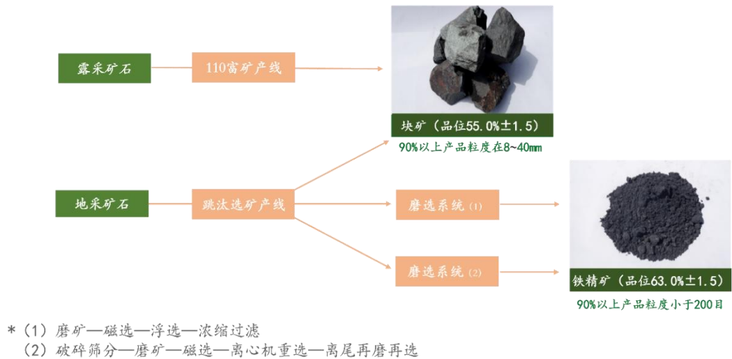
铁矿石产品生产流程图
