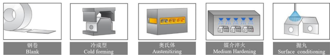
图：公司 MHP 工艺示意
