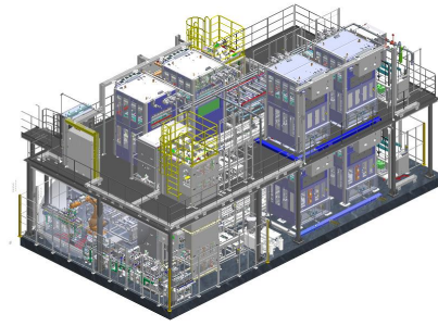
图:方腔式注液机
