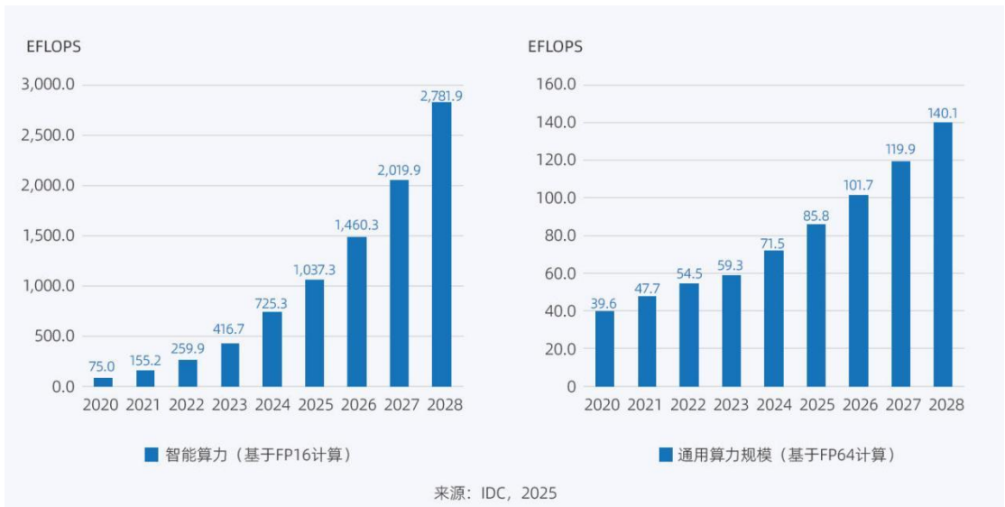
中国智能算力和通用算力规模及预测，2020-2028
