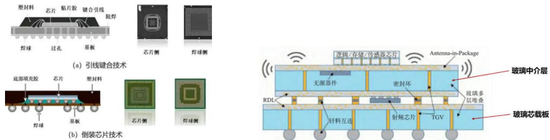
图：封装基板与芯片的常用互连技术及封装基板和玻璃基封装基板内部结构
