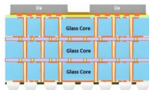
3D 先进封装(Chiplet)用全玻璃基载板结构示意图
