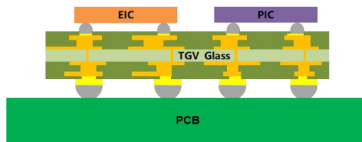
玻璃基 CP0 结构示意图
