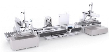
门锁加工连线
