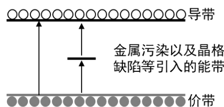
图：CIS 器件暗电流问题
