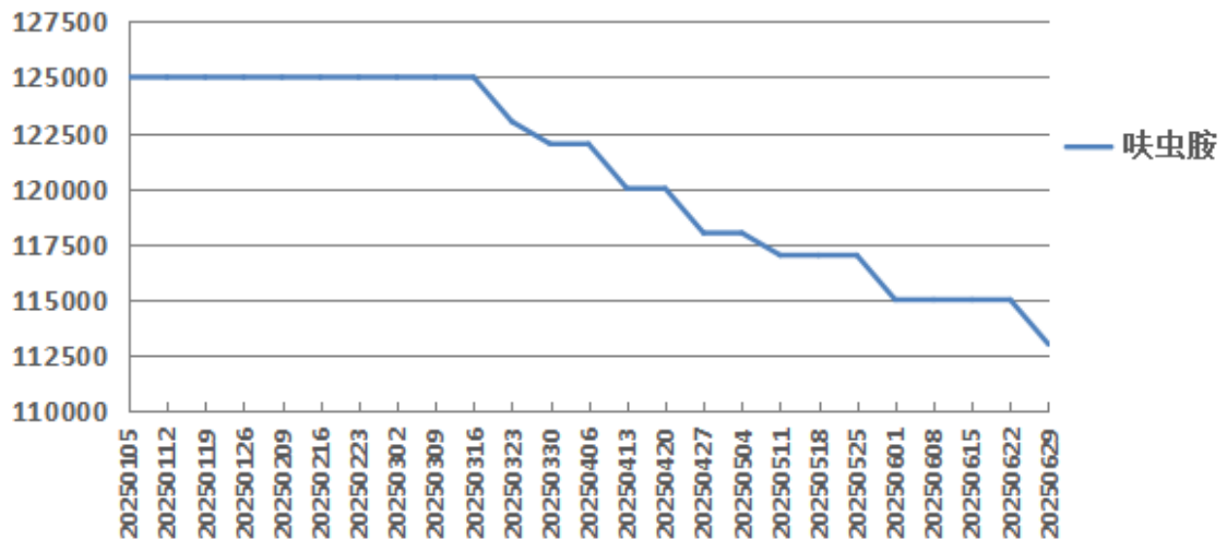
2025上半年呋虫胺原药价格走势图
