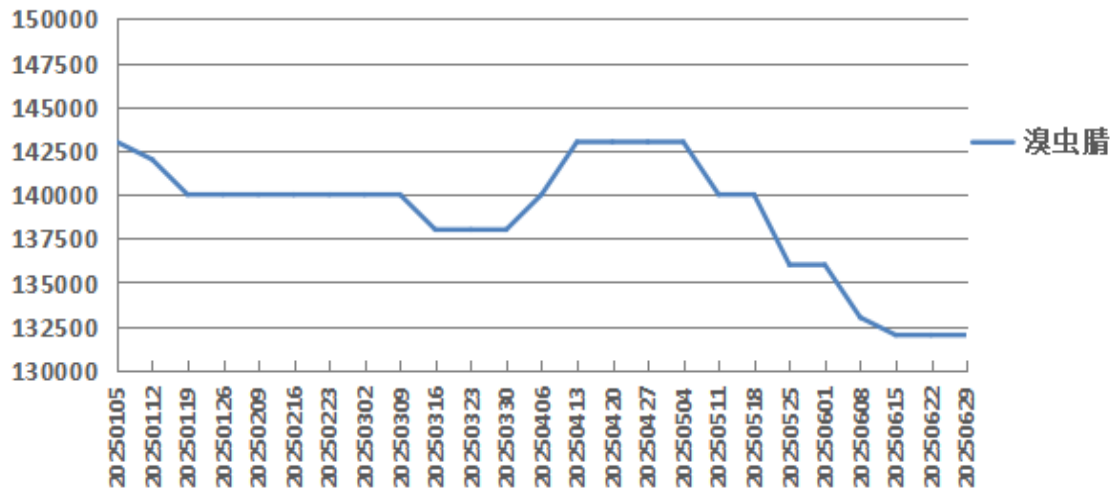
2025上半年溴虫腈原药价格走势图
